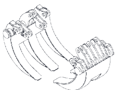
IMG H - Szczęki do manipulowania materiałem w układzie 3 + 2
